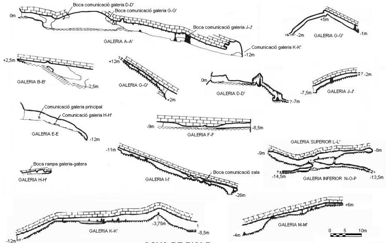
COVA DE RIALB Perfils traçats sobre la poligonal i rebatuts en un mateix pla
